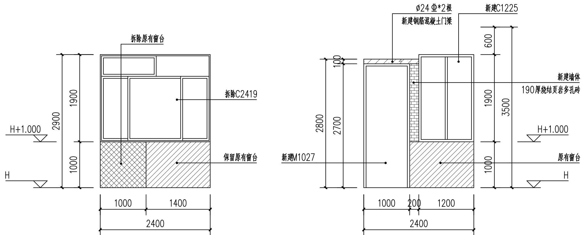
C 24 19拆除大样图 1:50
