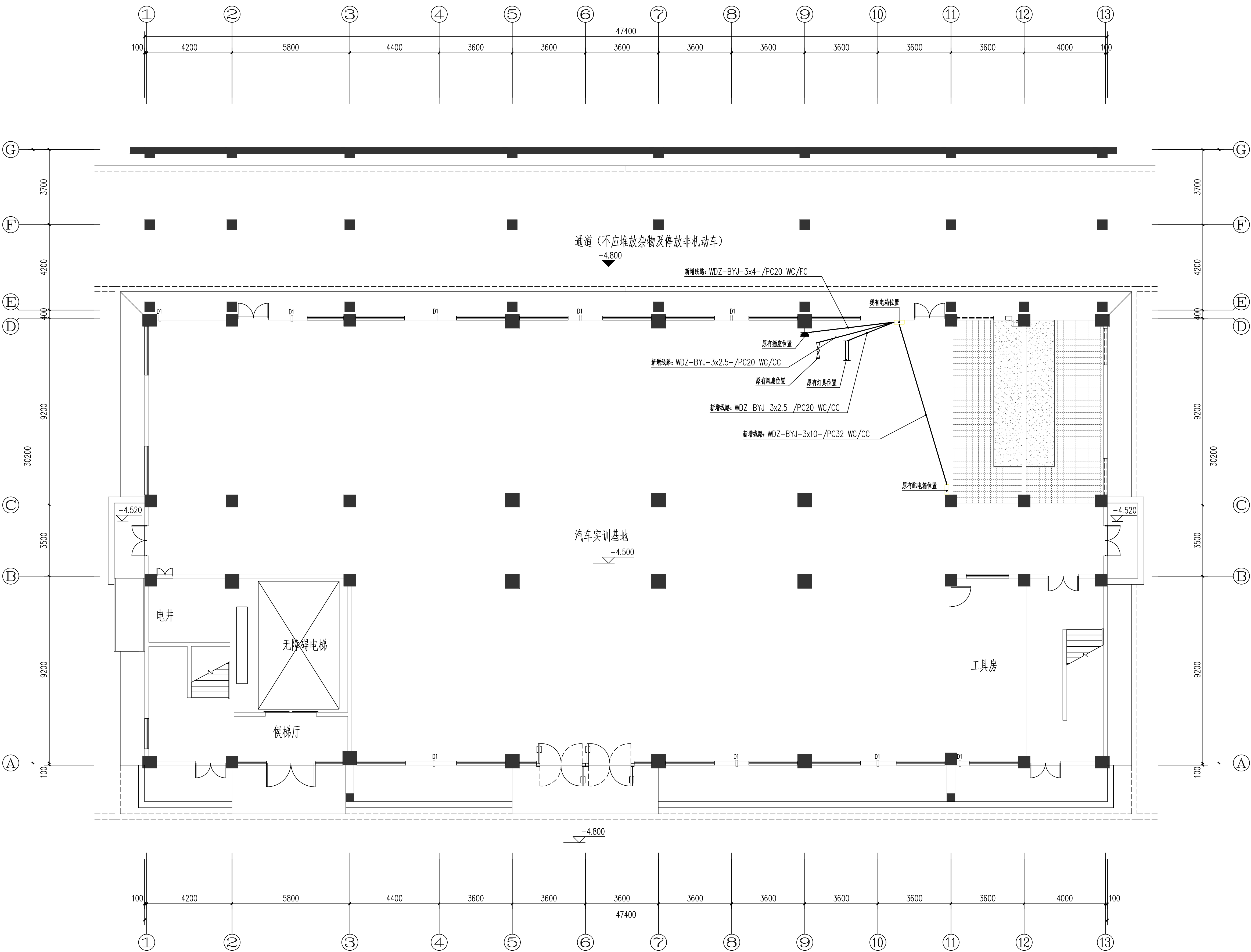
改造后一层电气平面图 1:100
