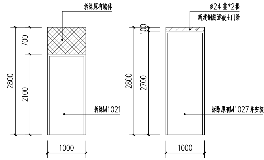
M2021更换为M1027大样图 1:50
