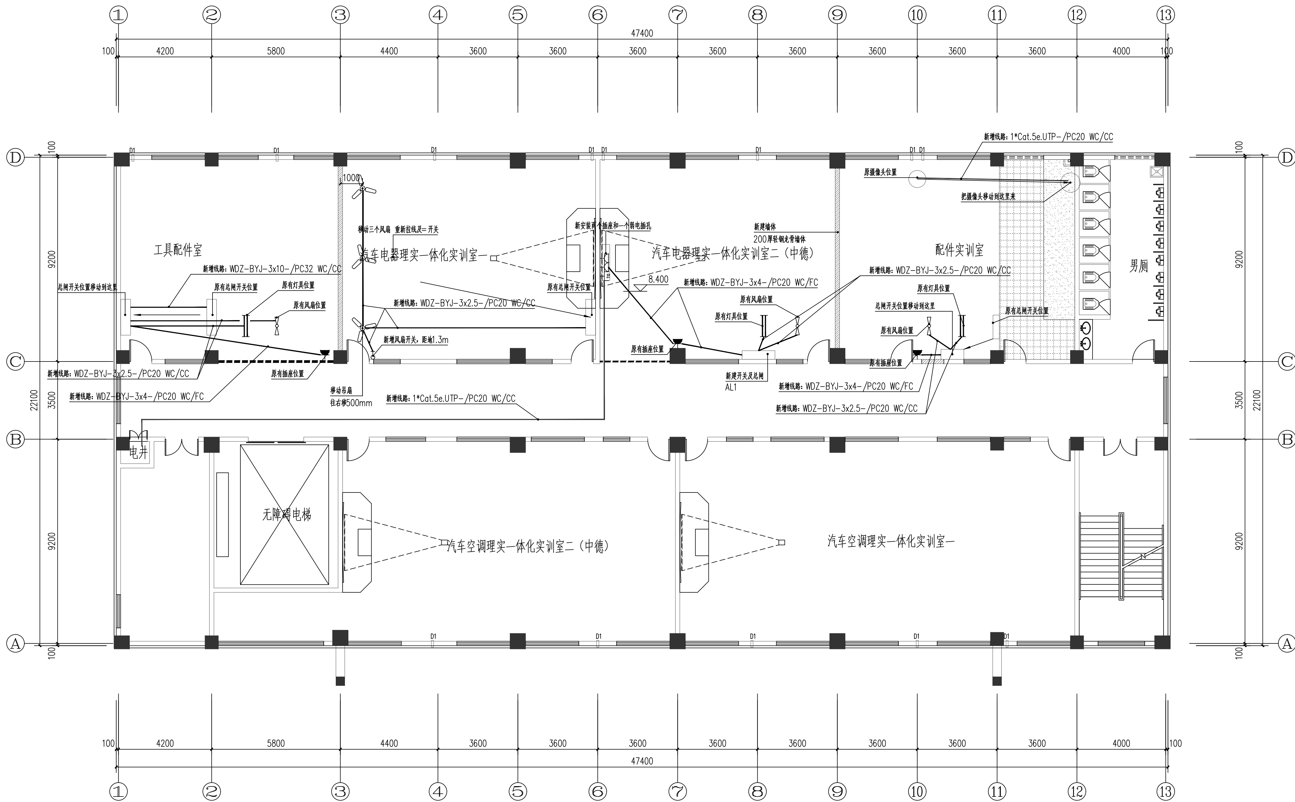
改造后四层电气平面图 1:100
