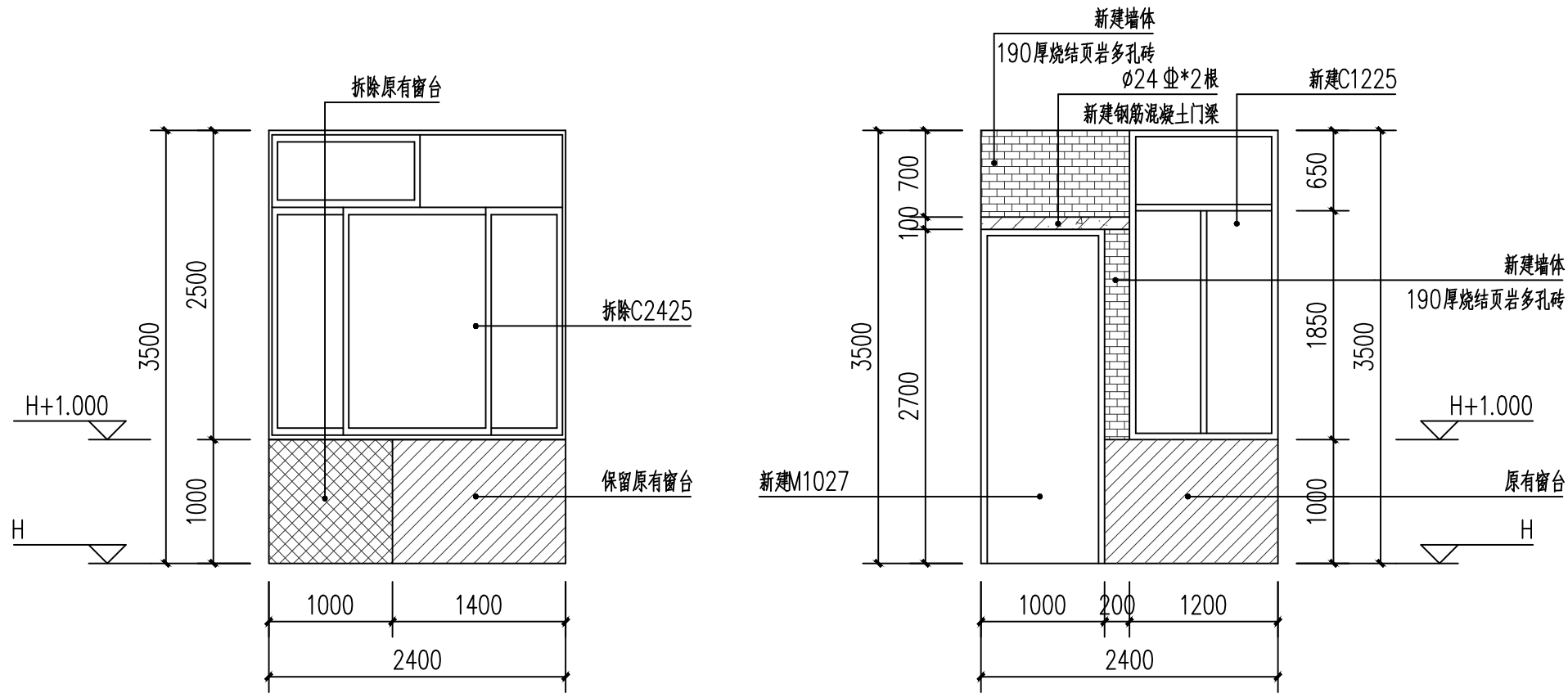
C 24 25拆除大样图 1:50
