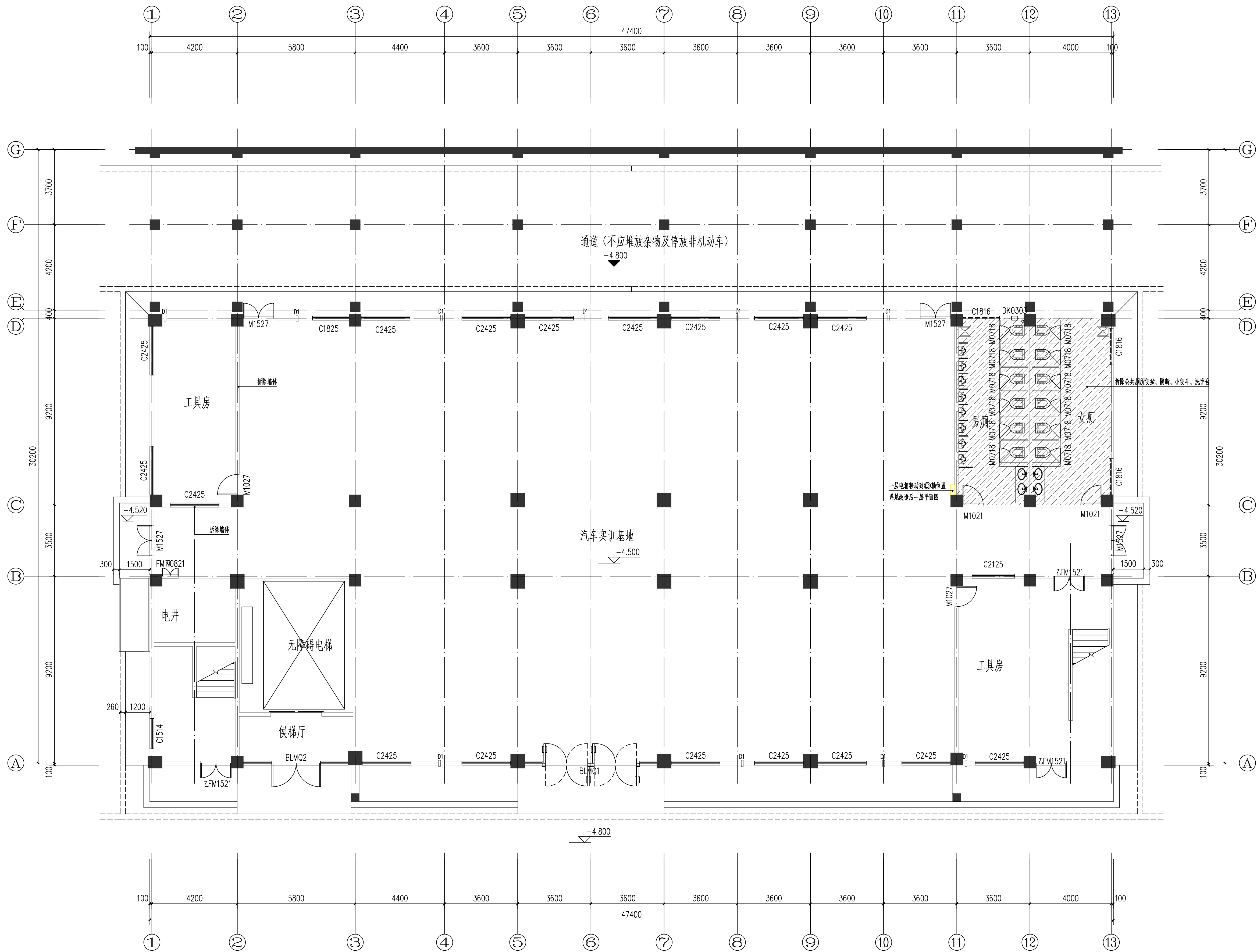
改造前一层平面图 1:100
