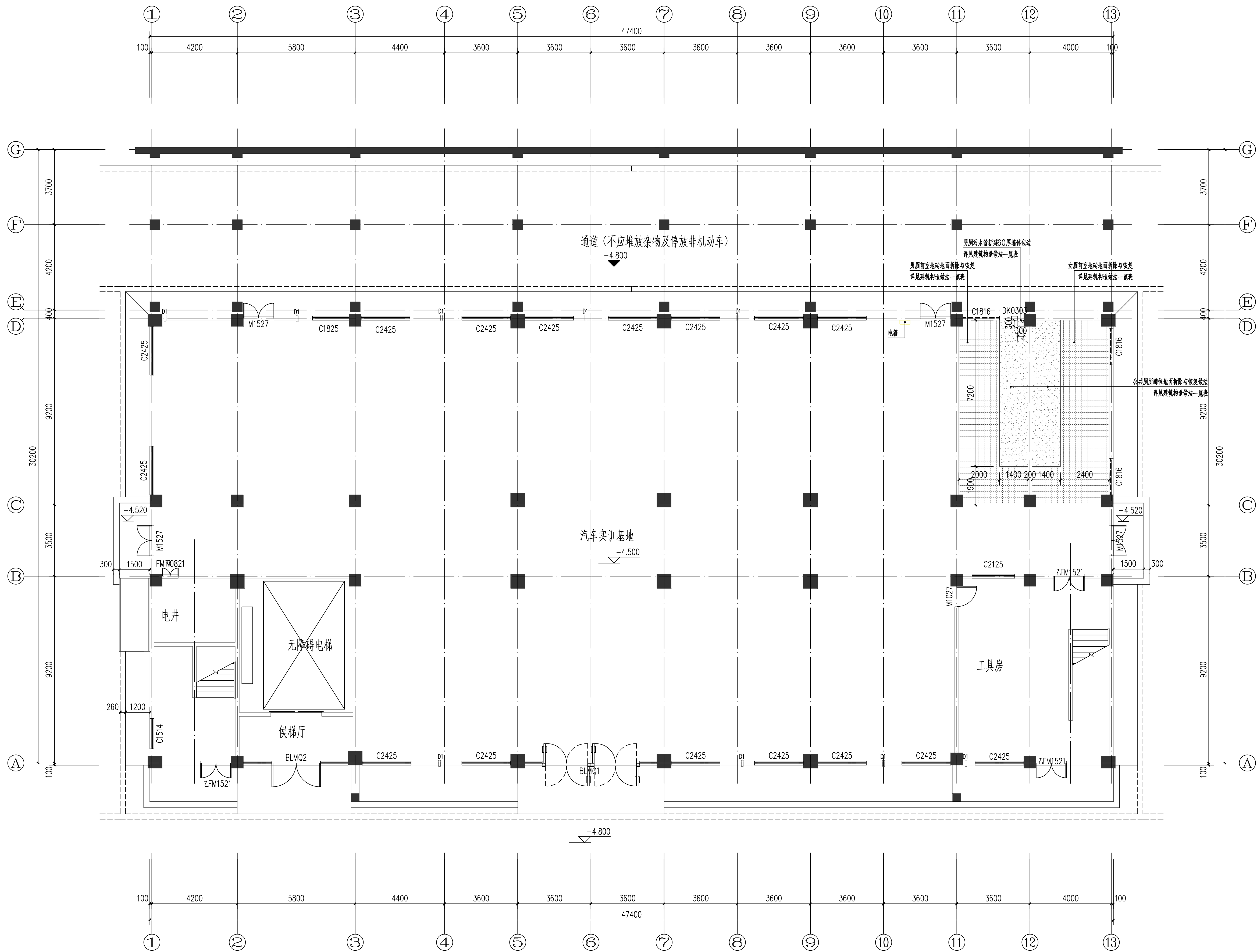
改造后一层平面图 1:100
