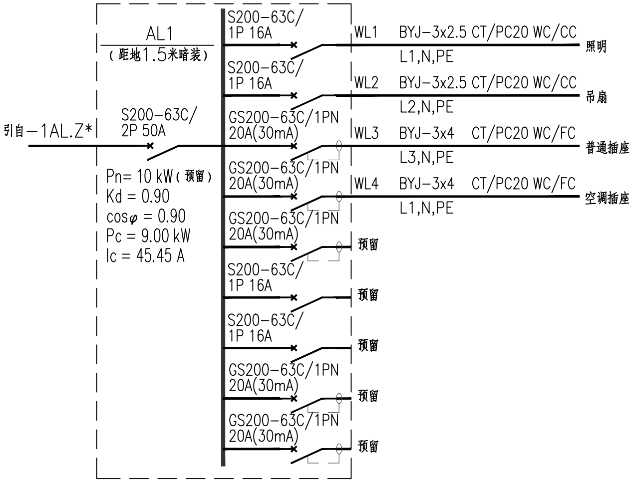
新增配电箱系统图
